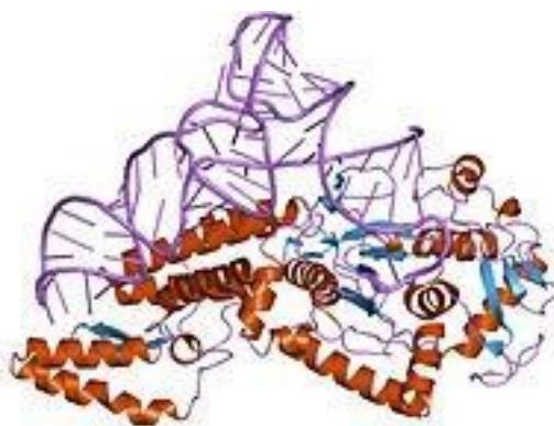
Slika 13. amonoacil-tRNA- sintetaza [30].
