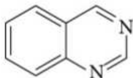
Slika 11. Kinazolin [12][13]
