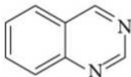
Slika 11. Kinazolin [12][13]
