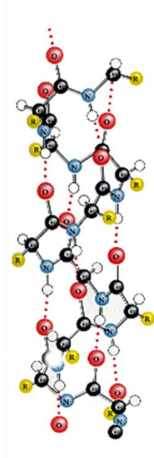
Slika 13. Prikaz \alpha -uzvojnice.
