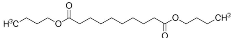
Slika 24. Struktura dibutil sebacata
