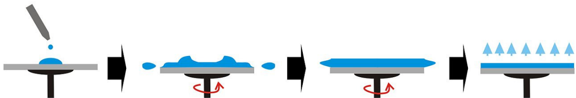
Slika 2.10. Spin-coating tehnika [35].
