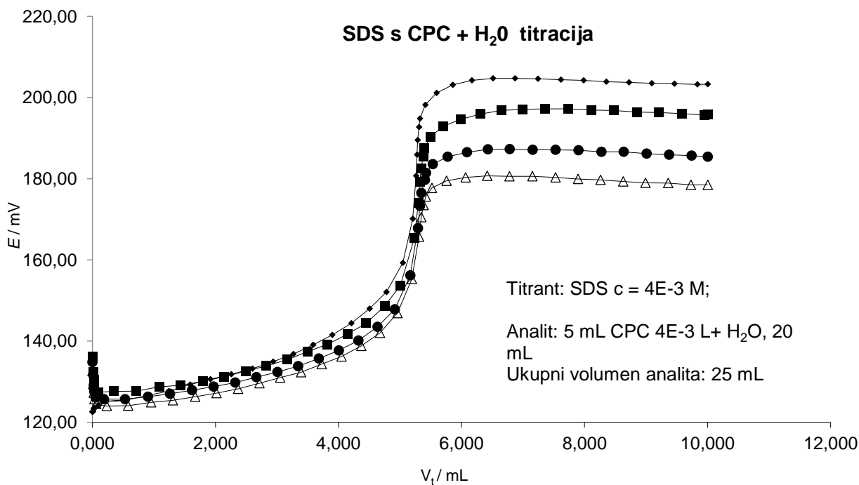
SLIKA 13. Titracija anionskog tenzida SDS s kationskim tenzidom CPC.
