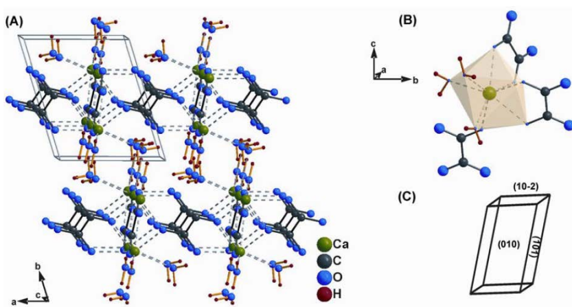
Slika 7. Kristalna struktura COT^{[10]} (A) i poliedar Ca^{2+} (B)
