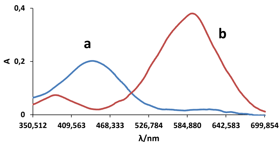
Slika 4.11. UV-Vis apсорpcijski spektar K12 senzorskog sloja na staklu u (a) kiselom mediju i (b) lužnatom mediju.
