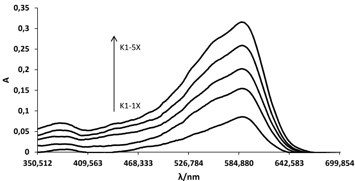
Slika 4.5. UV-Vis apsorpcijski spektri K1 senzorskih slojeva različitih sadržaja indikatora na staklu u lužnatom mediju.
