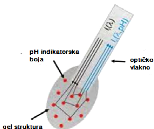
2.12. Shema optičkog sol-gel senzora za određivanje pH [45].
