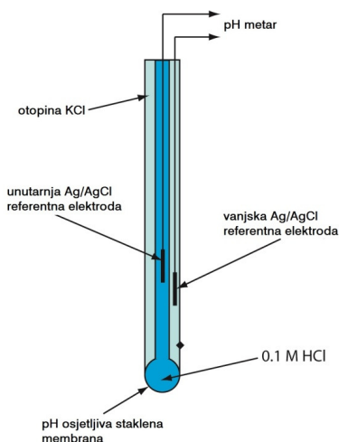
Slika 2.3. Staklena pH elektroda [12].
