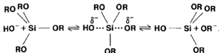
Slika 2.5. Mehanizam bazno-katalizirane hidrolize tetraalkoksisilana [14].
