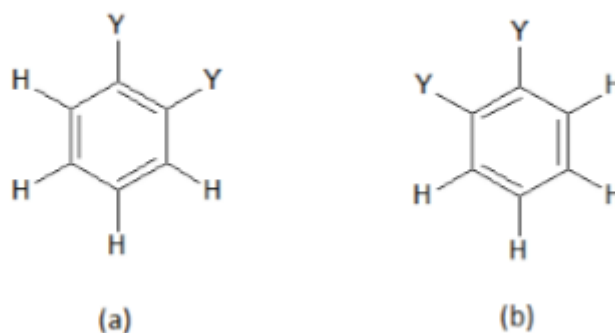
Slika 2.6.2.4. Orto-izomeri benzena
