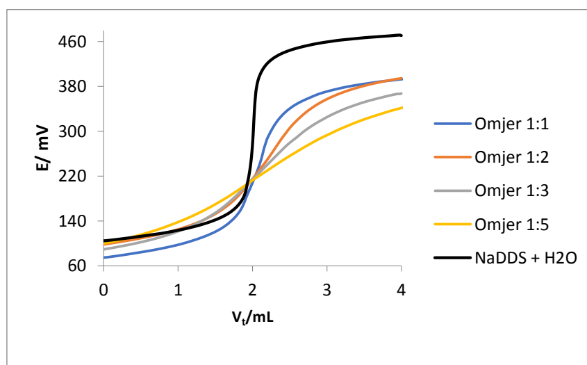
Slika 15. Prikaz titracijskih krivulja NaDDS-a, c = 4 \times 10^{-3} M, sa CPC-om, c = 4 \times 10^{-3} M, uz dodatak Genapola T150, c = 1 \times 10^{-2} M, u različitim molarnim omjerima u odnosu na NaDDS
