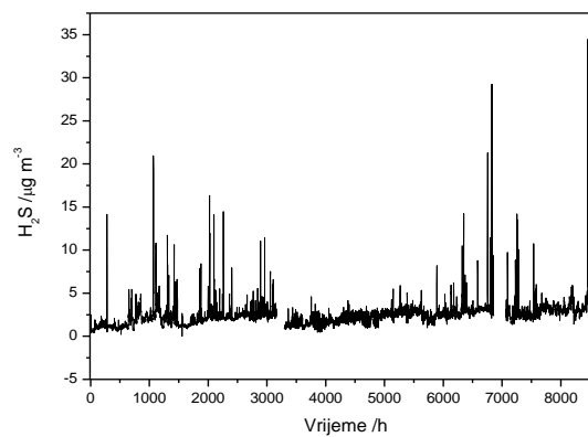
b) H 2 S
