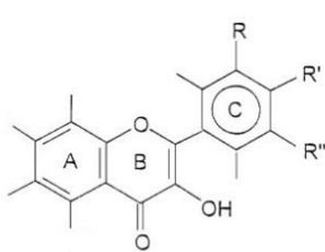
Slika 2. Flavonol
