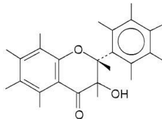
Slika 3. Flavanol
