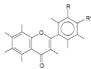
Slika 4. Flavon
