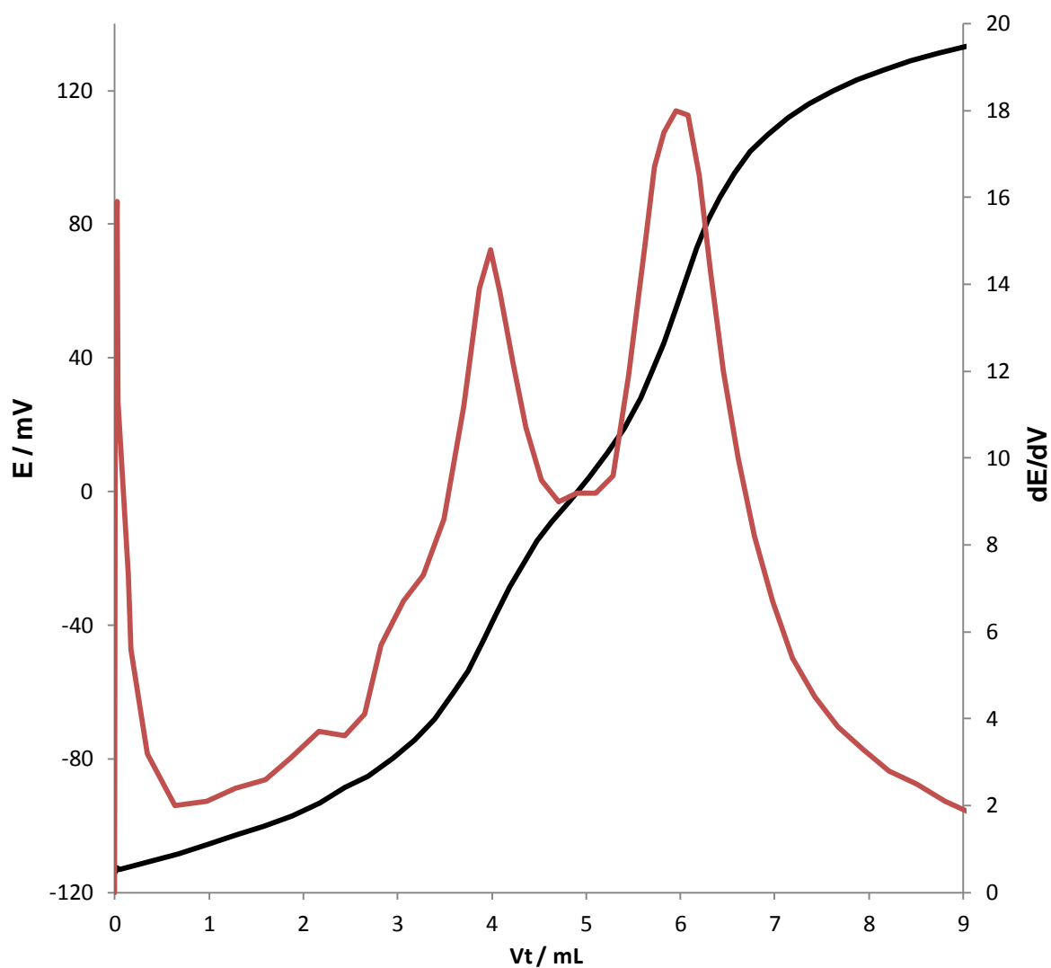
Slika 9. Krivulja potenciometrijske titracije smjese C_{10} i C_{12} s CPC koncentracije 1 \times 10^{-3} mol/dm 3 i njena prva derivacija
