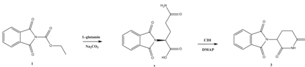
Slika 3. Sinteza talidomida [6]
