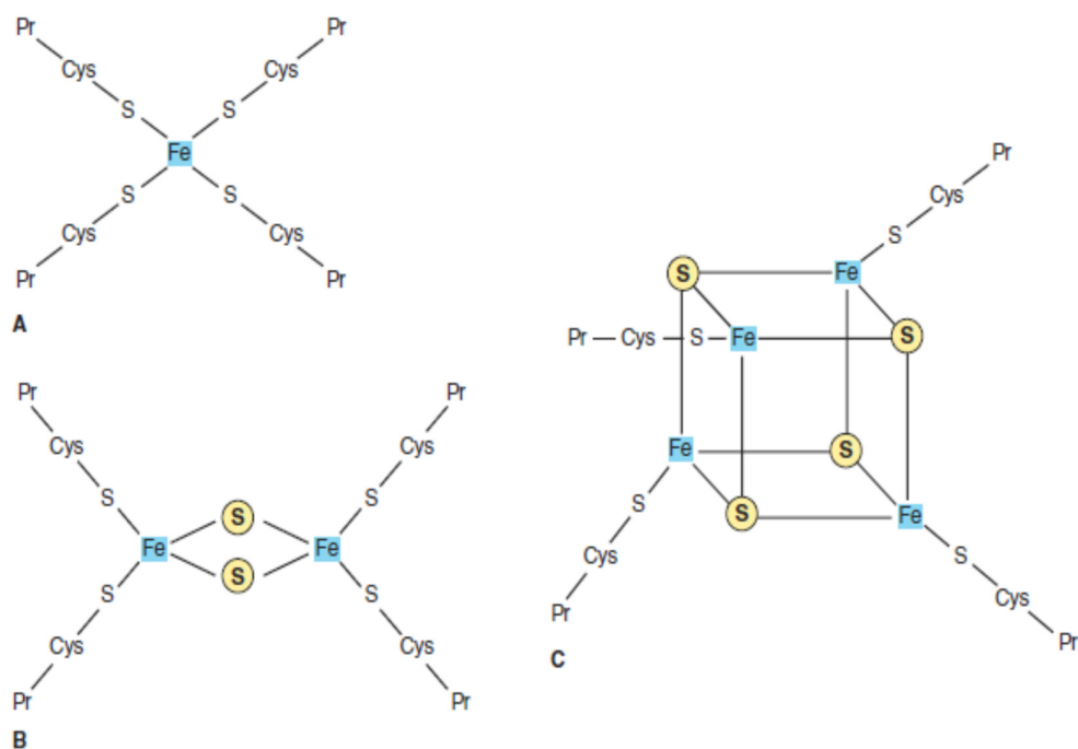
Slika 6. Klasteri željezo-sumpor.
