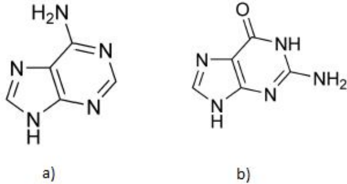
Slika 3. Purinske baze (adenin (a) i gvanin (b)) [4]
