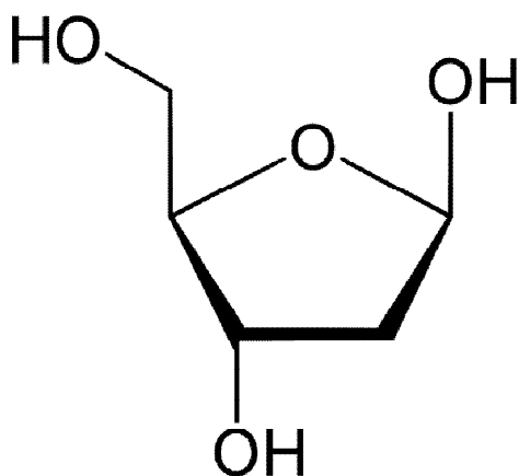
Slika 2. Šećer deoksiriboza
