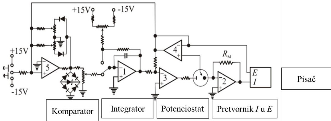
Shema 3. Uređaj za voltmetriju [15].
