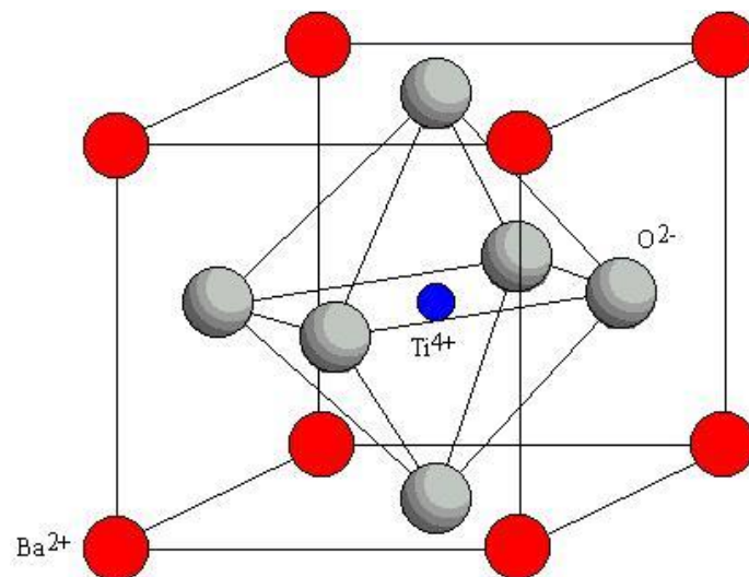
Slika 1. Struktura jednostavnog perovskita BaTiO_3 .
