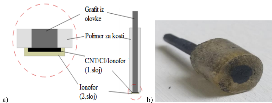
Slika 22. A) Shematski prikaz i; b) fotografija izrađenog CNTSS senzora.
