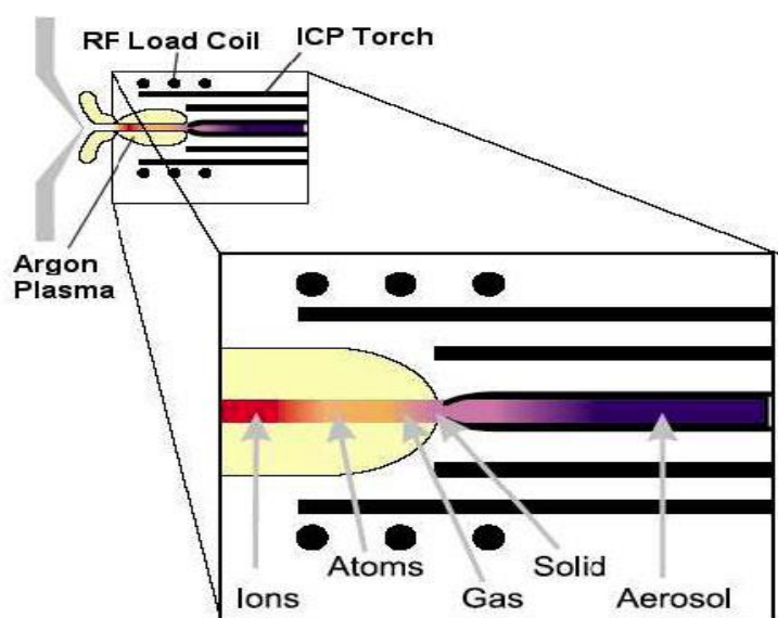
Slika 2. ICP plamenik [5]
