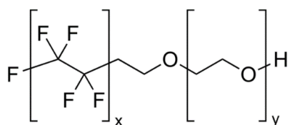
Slika 23. Struktura Zonyla [65]
