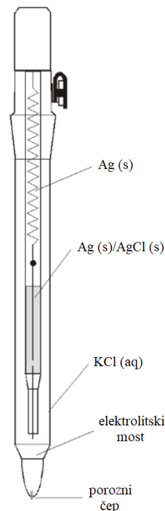
Slika 11. \text{Ag}/\text{AgCl} elektroda [23]
