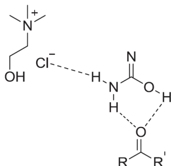
Slika 7. Formiranje vodikove veze između karbonilnog spoja i eutektičke smjese ChCl/U [18]
