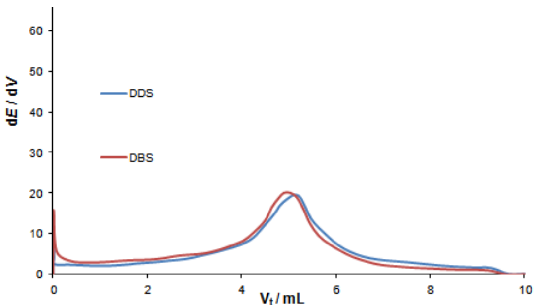
Slika 11: Derivacijske krivulje ( \Delta E / \Delta V ) za određivanje točke ekvivalencije pri potencimetrijskoj titraciji otopine NaDDS-a, c=1 \times 10^{-4} \text{ mol/dm}^3 i NaDBS-a, c=1 \times 10^{-4} \text{ mol/dm}^3 s otopinom CPC-a, c=1 \times 10^{-4} \text{ mol/dm}^3
