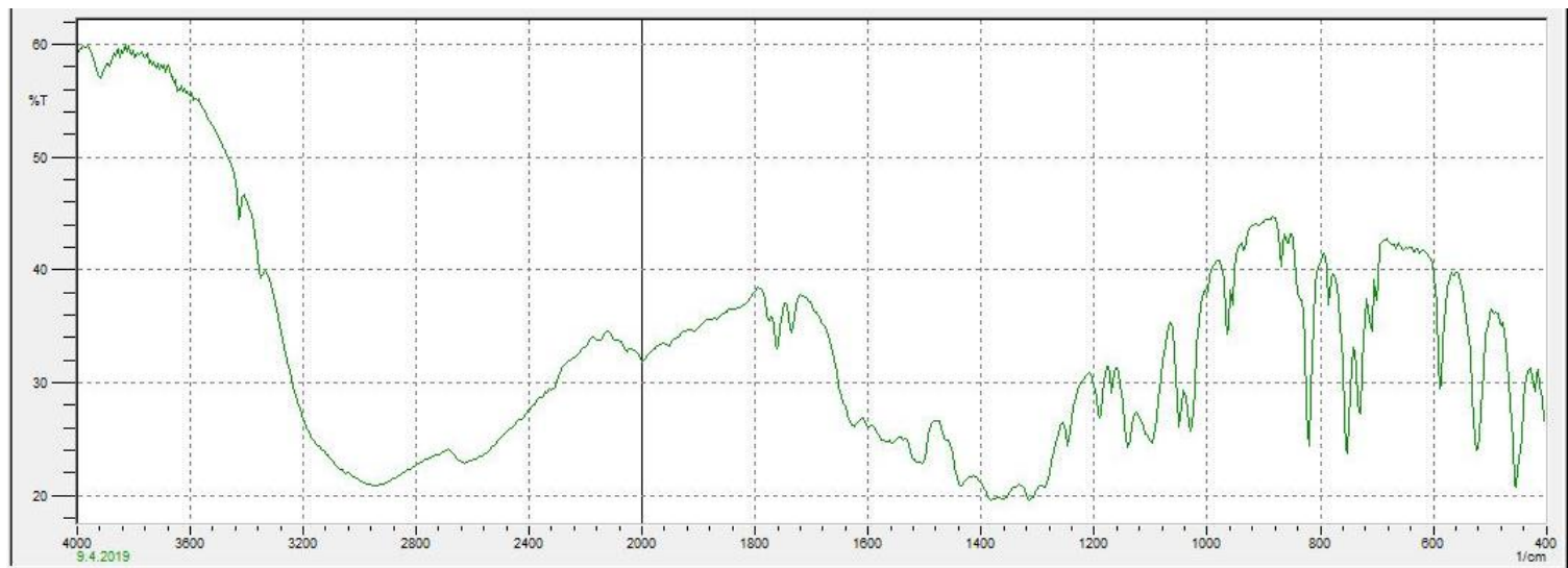
Slika 8. IR spektar o -fenilendinitrata
