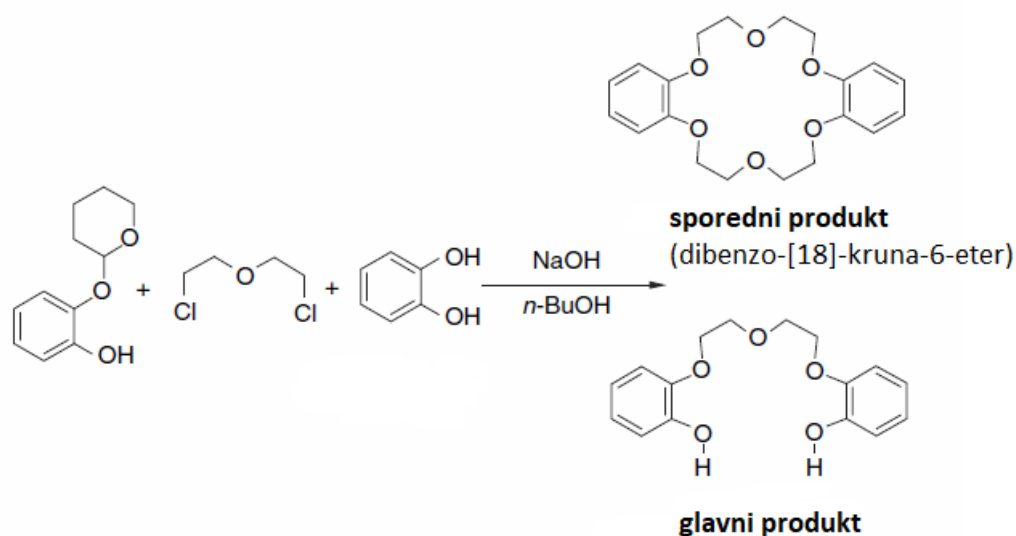
Slika 4. Charles J. Pedersen je slučajno otkrio dibenzo-[18]-kruna-6-eter (18-člani prsten s 6 donora atoma kisika) dobiven kao sporedni produkt prilikom pokušaja priprave bis(fenol) derivata zbog alkalne baze u tragovima koja je sadržavala metal 11
