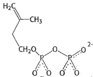
Slika 4.: 3-izopentenil-pirofosfat [2]
