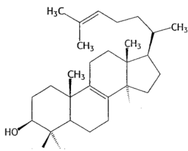
Slika 9.: Lanosterol [2]
