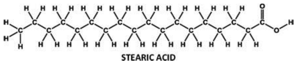
Slika 9. Stearinska kiselina
