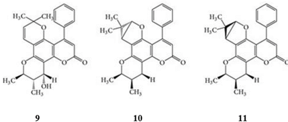
Slika 19: Strukture inofiluma
