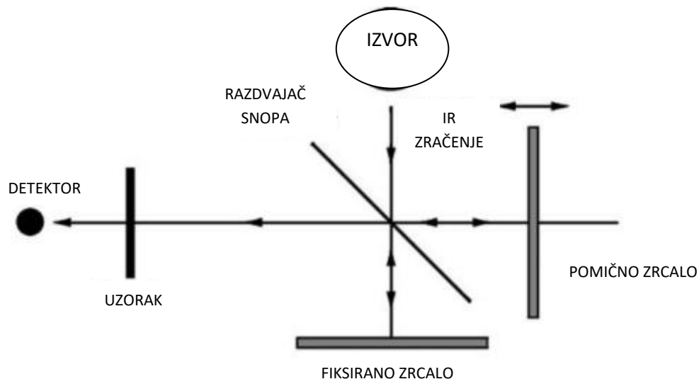
Slika 9. Shema FTIR-a [38]
