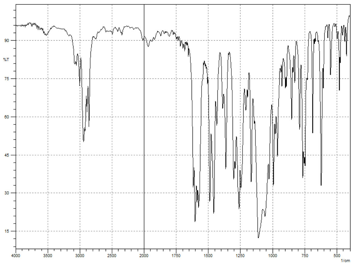
Slika 26. IR spektar spoja \text{AgLiClO}_4
