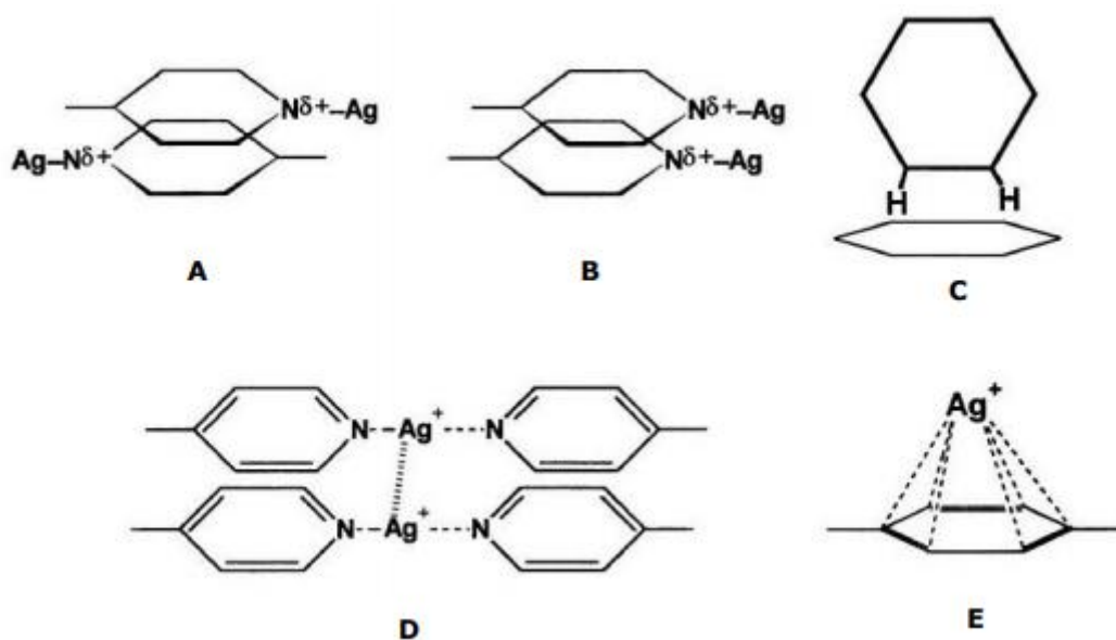
Slika 11. Shematski prikaz supramolekulskih veza između aromatskih prstenova u kompleksnim spojevima. a) glava-rep, b) glava-glava, c) rub-glava, d) metal-metal interakcija, e) interakcija \text{Ag(I)} -kationa s \pi -elektronom aromatskog prstena [16].
