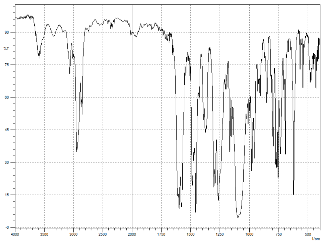
Slika 27. IR spektar spoja \text{AgL}_2\text{ClO}_4
