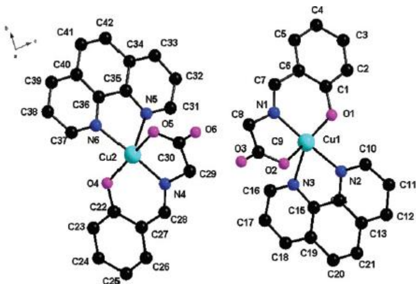
Slika 6. Kristalna struktura Cu-1,10-fenantrolina, preuzeto iz [27].
