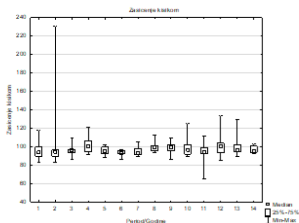
Slika 79. Grafički prikaz rezultata Kruskal-Wallis testa primjenjenog na podatke zasićenja kisika, rijeke Drave ( \text{mgO}_2/\text{dm}^3 ) u vremenskom periodu 2004.-2017.
