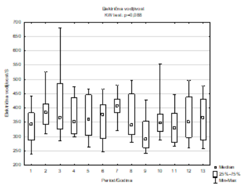
Slika 64. Grafički prikaz rezultata Kruskal-Wallis testa primjenjenog na podatke električne vodljivosti rijeke Drave u vremenskom periodu 2004.-2017.
