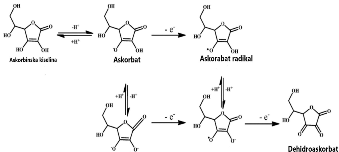
Slika 1. Mehanizam uklanjanja radikala askorbinske kiseline; prilagođeno iz [3]
