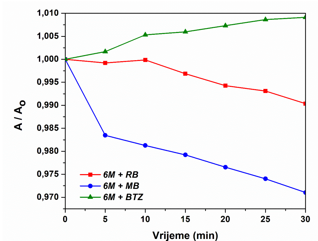
Slika 28. Ovisnost promjene apsorbancije ( A/A_0 ) o vremenu za interakciju SMO_6M fotokatalizatora s rodaminom B, metilenom plavo i bromtiomolom zeleno.
