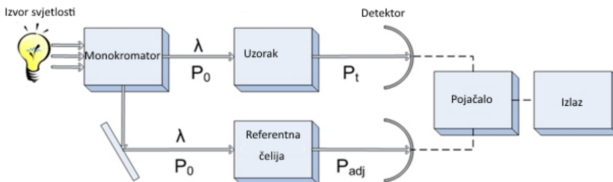
Slika 11. Shema dvosnognog spektrofotometra [22].
