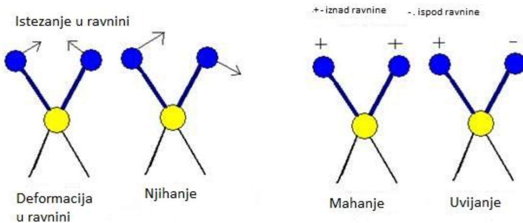
Slika 6. Prikaz vibracija deformacija molekule [16].
