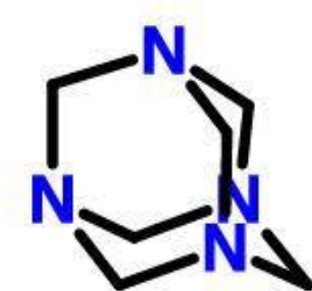
Slika 4. Struktura heksametilentetraamina [11].
