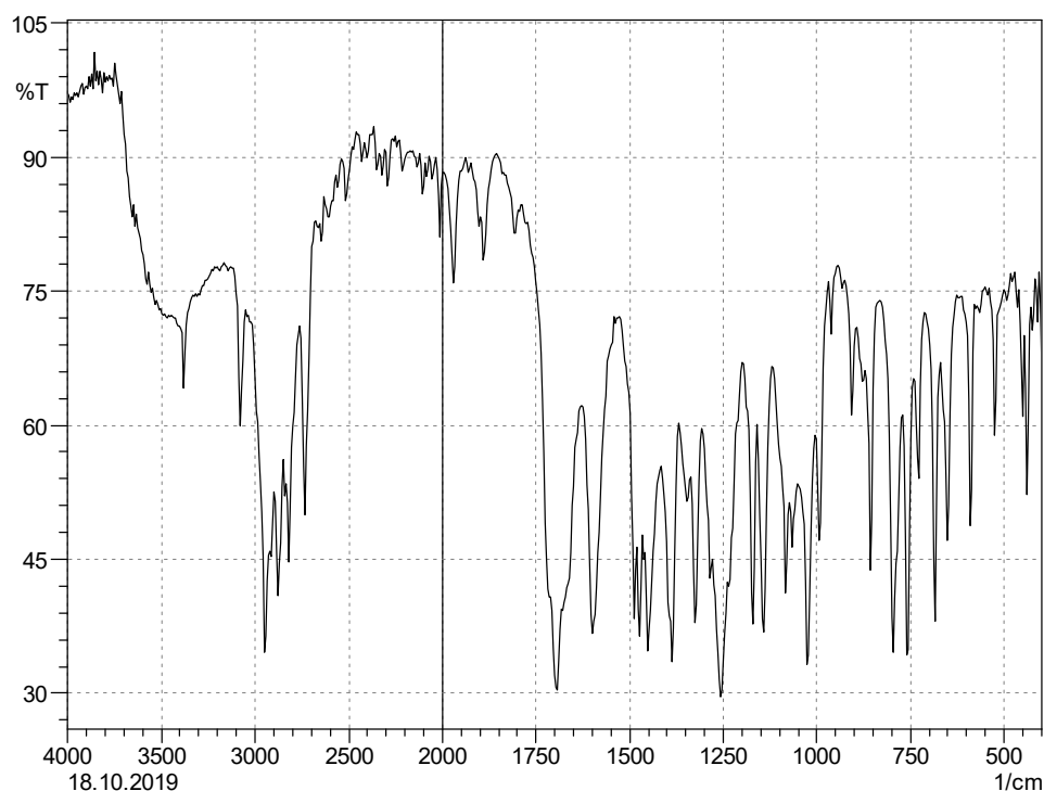
Slika 20. FTIR spoja 3
