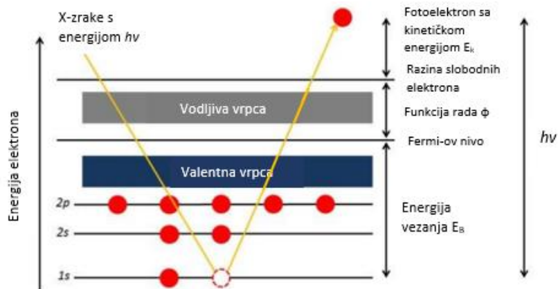
Slika 34. Fotoelektrični efekt [75].
