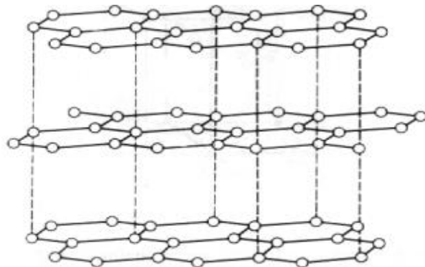
Slika 2. Struktura grafita [3]
