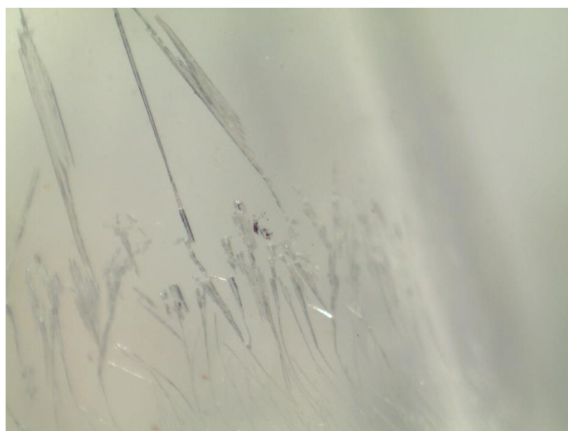
Slika 35. Igličasto/pločasti kristali spoja Do3OH pripravljeni metodom evaporacije uz otapalo metanol
