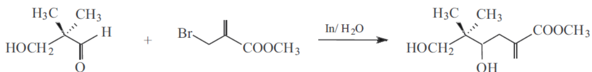
Slika 3. Reakcija kopulacije katalizirana indijem
