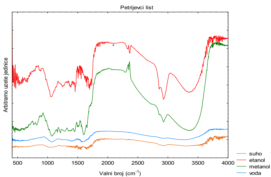
Slika 16. FTIR spektri listova imele s područja Petrijevaca (etanol, metanol i voda u usporedbi sa suhim uzorkom)
