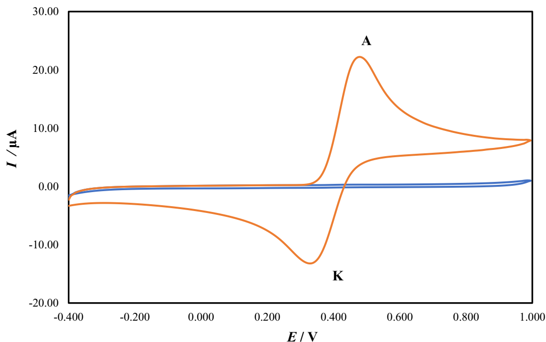
Slika 15. Ciklički voltamogrami blank otopine (pufer pH = 4) (—) i otopine 3,4-dihidroksibenzojeve kiseline (—) ( c = 1 \cdot 10^{-3} \text{ mol/dm}^3 ), \nu = 50 \text{ mV/s} .
