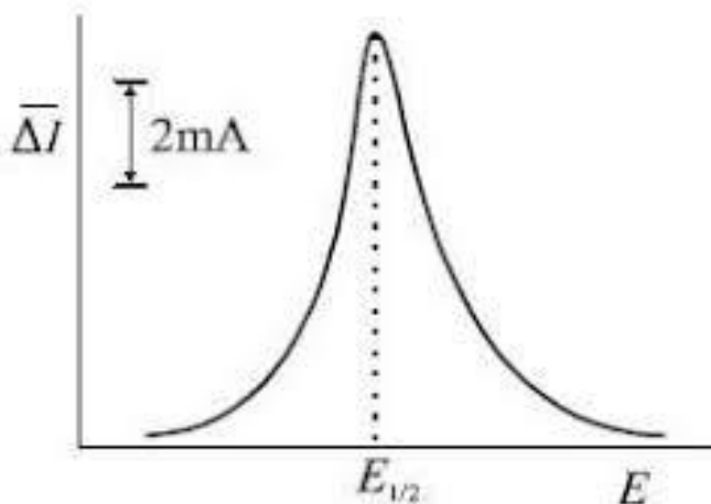
Slika 11. Signal odziva kod diferencijalne pulsne voltametrije [28].
