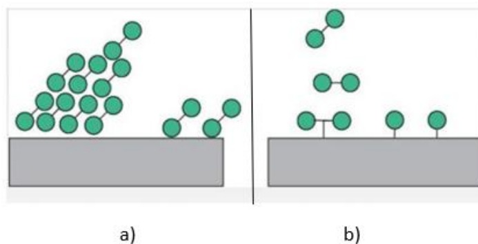
Slika 9. Prikaz polimolekularnog sloja (a) i monomolekularnog sloja (b).
