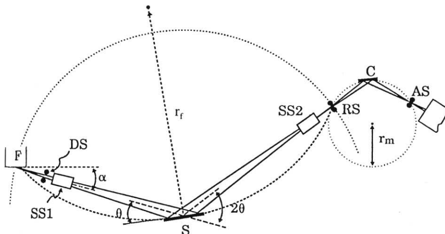
Slika 11. Bragg-Brentano difraktometar [36].
