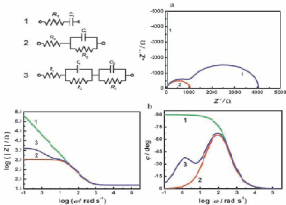
Slika 5. Grafički prikaz simuliranih IS-a za dane EEC-e u: a) kompleksnoj ravni impedancije i b) Bodeovu prikazu. Vrijednosti parametara su: R_1 = 50 \Omega , C_1 = 5 \cdot 10^{-5} F , R_2 = 1000 \Omega , C_2 = 5 \cdot 10^{-4} F , R_3 = 3000 \Omega
