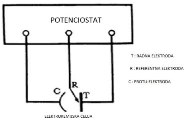
Slika 15. Potenciostat.
