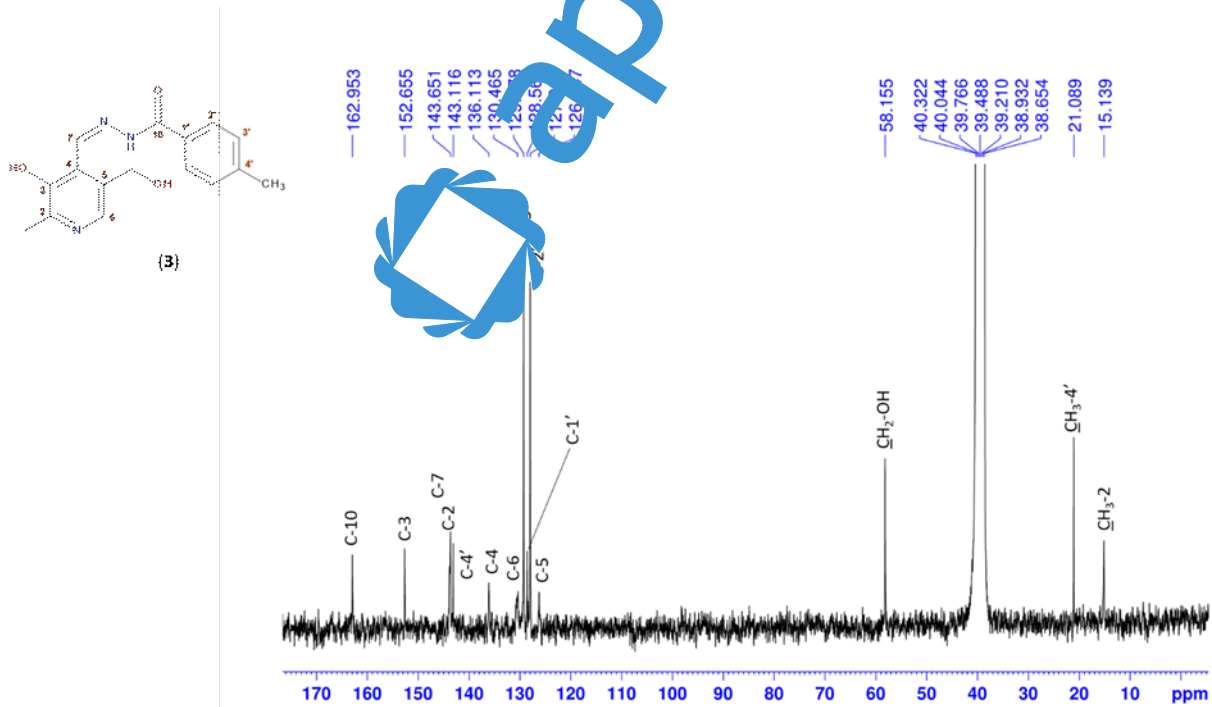
Slika 28. 13 C spektar N'-((3-hidroksi-5-(hidroksimetil)-2-metilpiridin-4-il)metilen)-3-metilbenzohidrazida (3)
