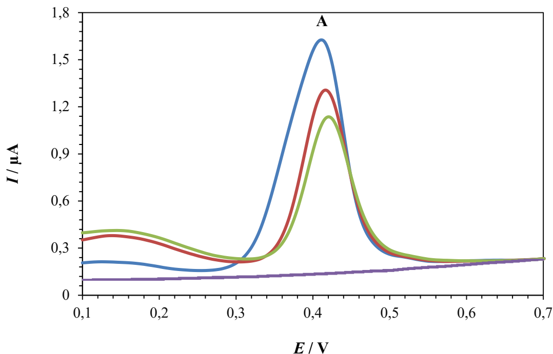
Slika 24. Diferencijalni pulsni voltamogrami blank otopine (pufer pH=5) (—) i uzastopno snimljene alkoholne otopine serotonina ( c=1 \cdot 10^{-4} mol \text{dm}^{-3} ) na elektrodi od staklastog ugljika, v=5 mV/s. (1. scan (—), 2. scan (—), 3. scan (—)) na elektrodi od staklastog ugljika u puferu pH=5.
