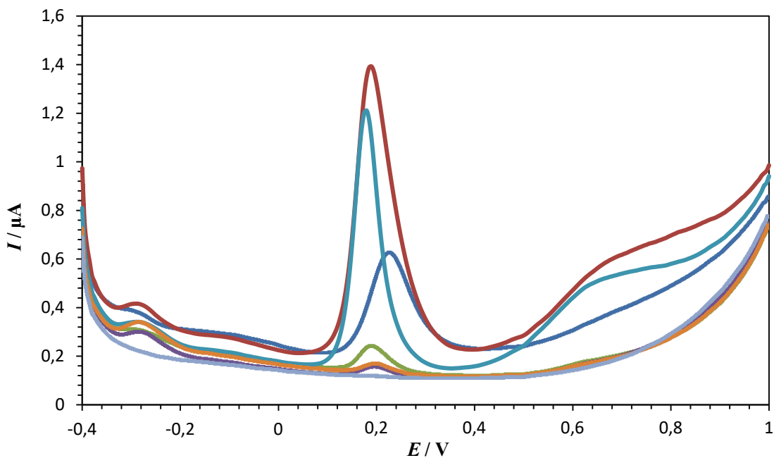
Slika 25. a) Diferencijalni pulsni voltamogrami blank otopine (pufer pH=9) ( \text{—} ) i alkoholnih otopina serotonina različitih koncentracija ( c=1 \cdot 10^{-6} ( \text{—} ), 5 \cdot 10^{-6} ( \text{—} ), 1 \cdot 10^{-5} ( \text{—} ), 5 \cdot 10^{-5} ( \text{—} ), 1 \cdot 10^{-4} ( \text{—} ), 1,4 \cdot 10^{-4} ( \text{—} ) mol \text{dm}^{-3} ) snimljeni na elektrodi od staklastog ugljika u puferu pH=9.
