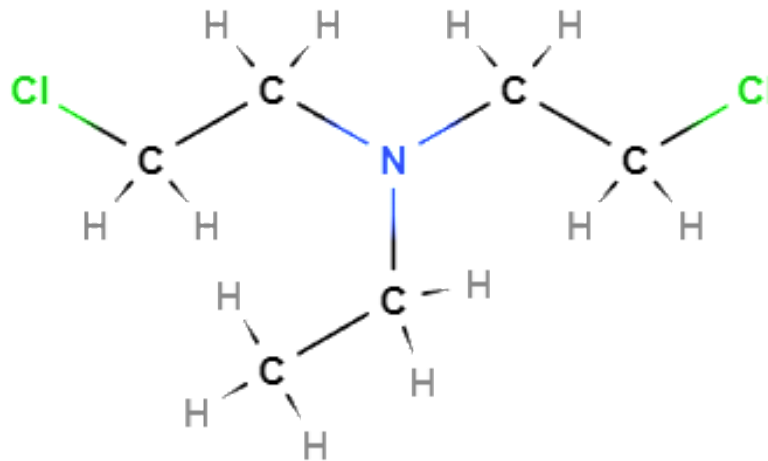
Slika 9. Struktura HN-1
