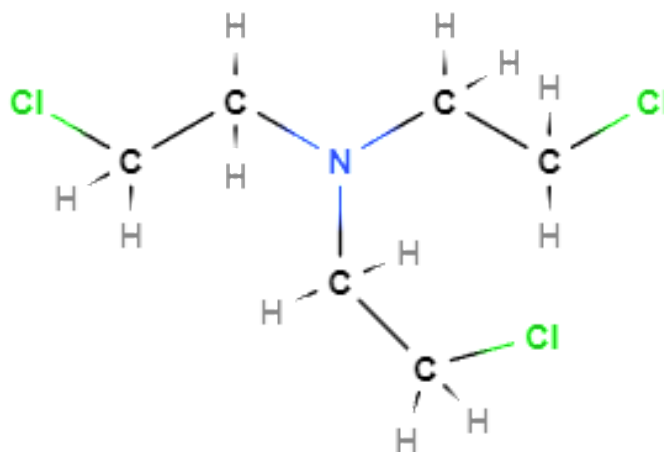
Slika 11. Struktura HN-3
