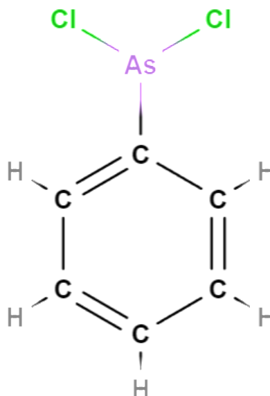
Slika 12. Struktura PD
